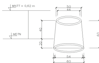
Hình 4: hình dạng và kết cấu bầu bê tông cốt xenlulo
